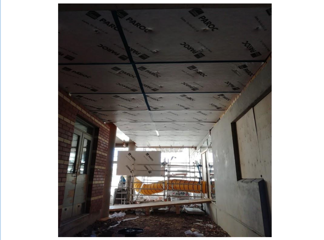
Kuva 4. Laajennus, pääsisäänkäynnin katoksen eristeiden asennus
