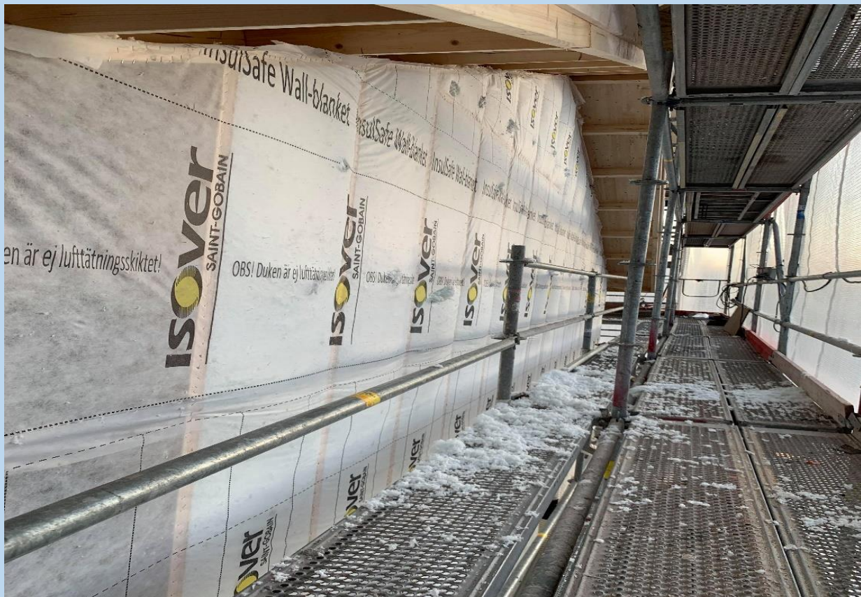
Kuva 2. Saneerausosan villanpuhallus.
